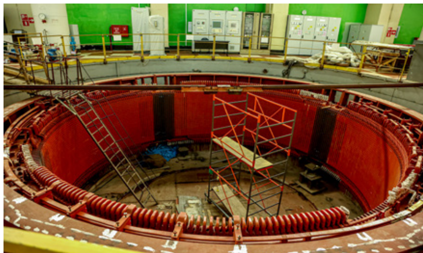
Обмотка гидрогенератора состоит из 4 секций, каждая из которых весит около 46 тонн
